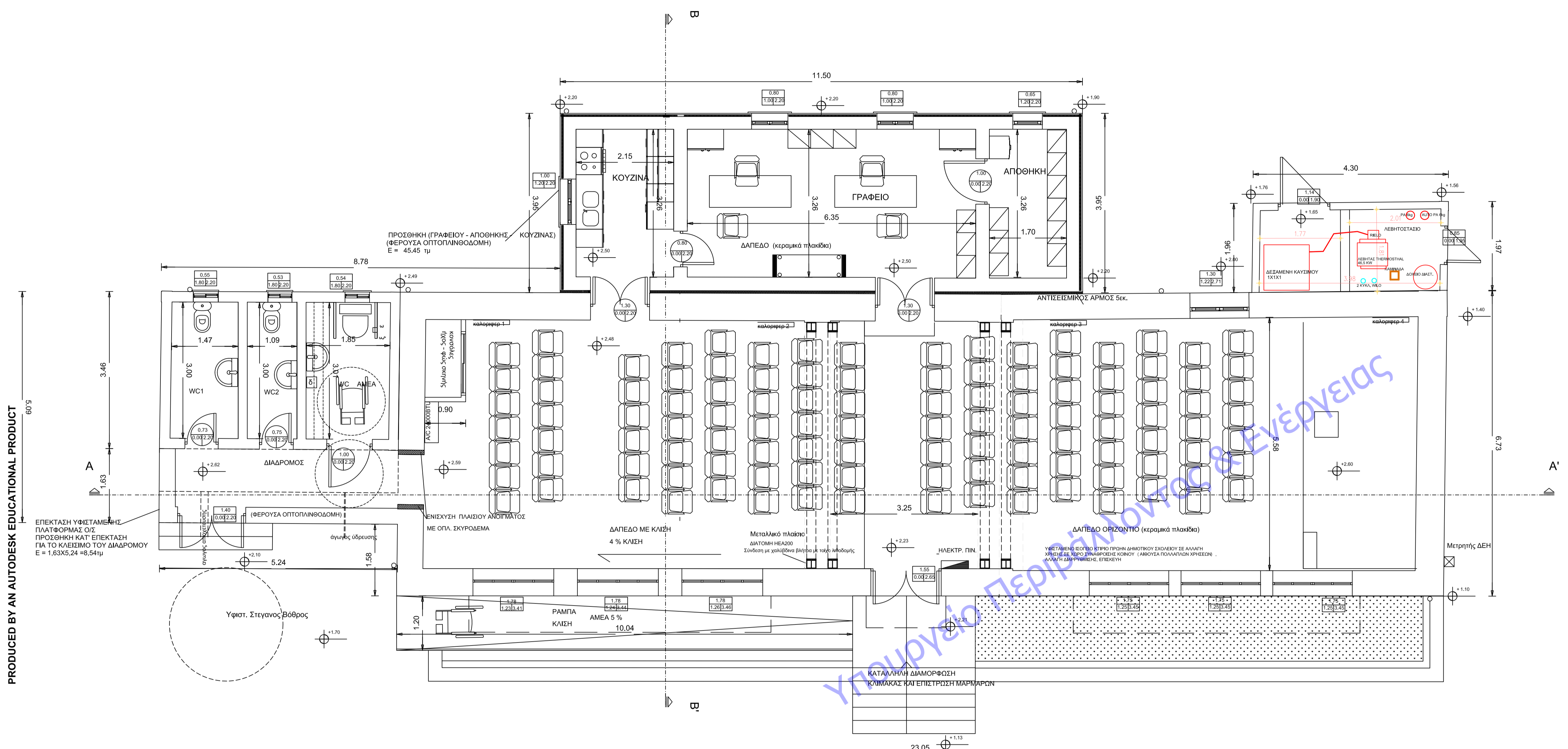
ΚΑΤΟΨΗ ΙΣΟΓΕΙΩΝ ΚΤΙΡΙΩΝ ΑΙΘΟΥΣΑΣ ΣΥΝΑΘΡΟΙΣΗΣ ΚΟΙΝΟΥ, ΧΩΡΩΝ ΥΓΙΕΙΝΗΣ, ΓΡΑΦΕΙΟΥ ΜΕ ΑΠΟΘΗΚΗ ΚΑΙ ΚΟΥΖΙΝΑΣ (ΠΡΟΤΑΣΗ)
